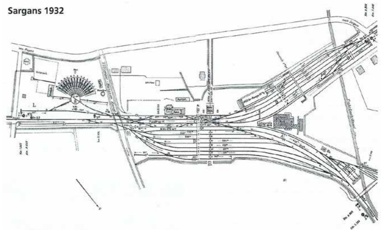
Der damals bauliche «Militärplan» des Bahnhofs Sargans vom Juni 1932 zeigt den Kilometer 0 und die Nutzlänge aller Gleisabschnitte. Zeichnung: SBB, Sammlung S. Niklaus
