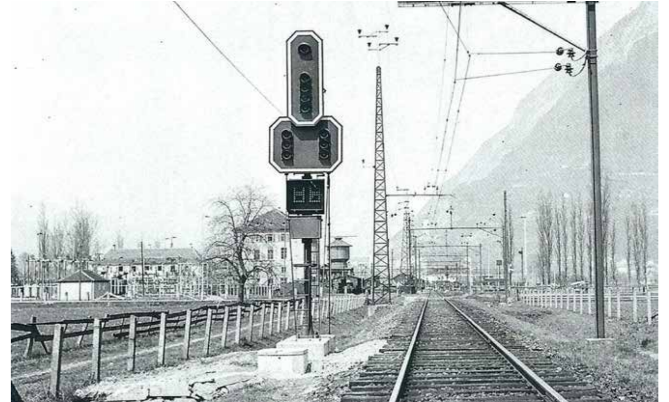
Damals fabrikneues Lichttagessignal Bauart Westinghouse als Einfahrsignal Seite Bad Ragaz, Durchfahrtsignal und Gleisnummernsignal. Ganz links das Unterwerk, in der Mitte der Wasserturm des Depots. 29.4.1938.
